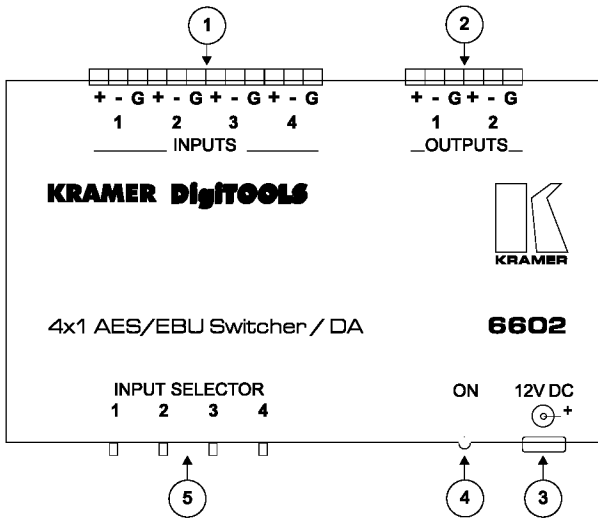
Figure 1: 6602 4x1 AES/EBU Switcher / DA
