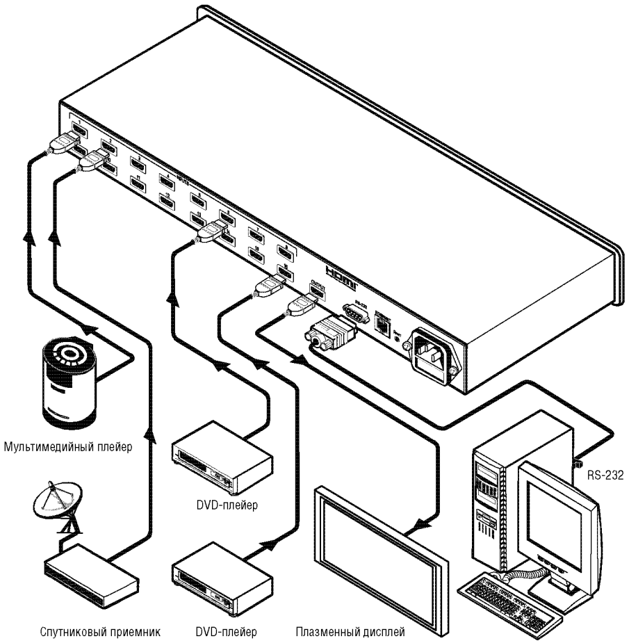
Рис. 2. Подключение источников и приемника сигнала к VS-161HDMI
