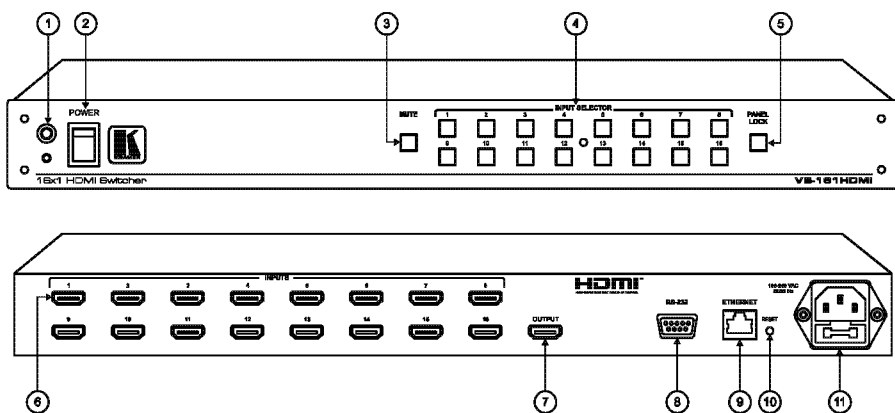
Рис. 1. Коммутатор VS-161HDMI
