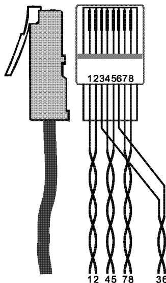
Рис. 4. Разводка кабеля на разъем RJ-45
