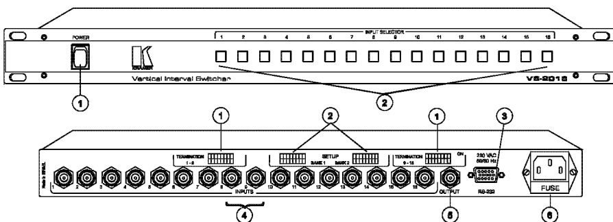
Рис. 1. Элементы передней и задней панели VS-2016
