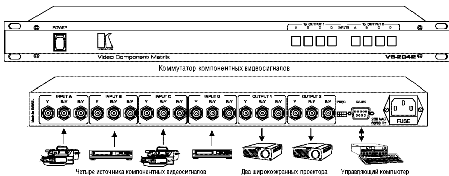
Рис. 9. Подключение матричного коммутатора компонентных видеосигналов для презентационных целей
