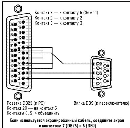
Рис. 1. Распайка разъема управления RS-232
