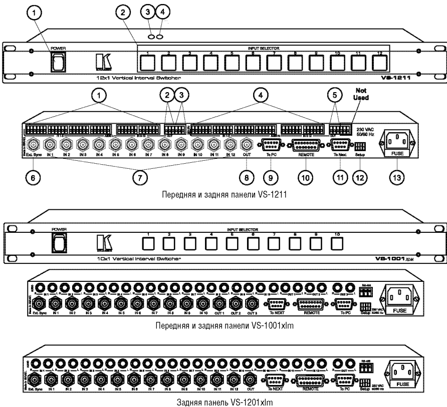
Рис. 2. Передняя и задняя панели VS-1011xlm/VS-1201xl
