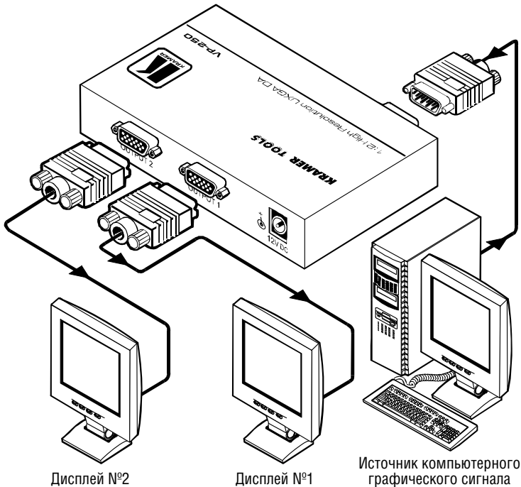
Рис. 4. Подключение источника и приемников сигнала к VP-250
