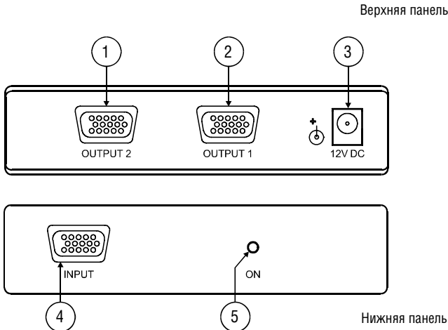
Рис. 2. Верхняя и нижняя панели VP-250
