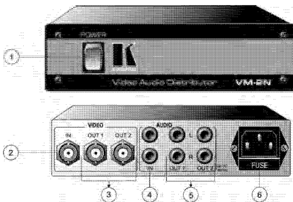
Рис. 1. Усилитель-распределитель VM-2N
