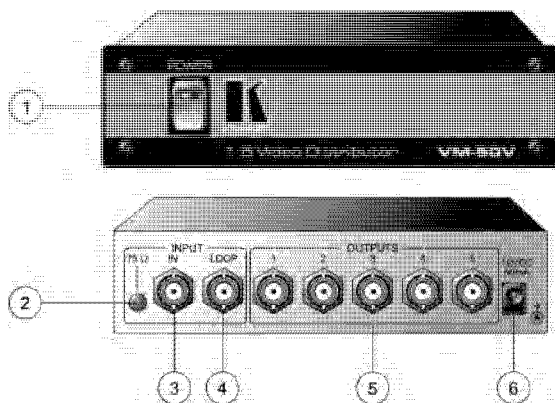
Рис. 6. Усилитель-распределитель VM-50V
