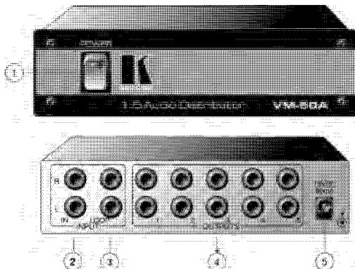
Рис. 3. Усилитель-распределитель VM-50A
