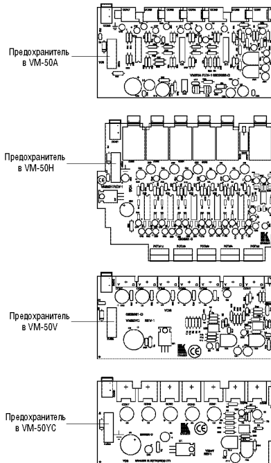
Рис. 9. Расположение внутреннего предохранителя
