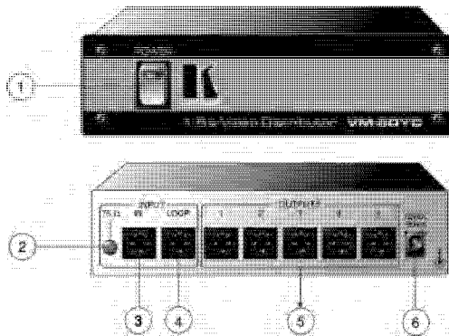
Рис. 5. Усилитель-распределитель VM-50YC
